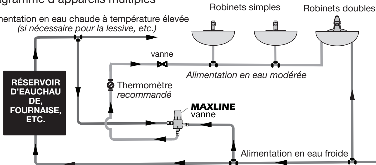
Diagramme d'appareils multiples
