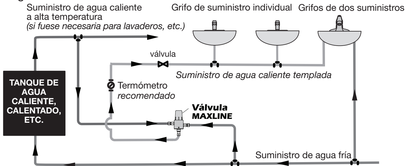
Diagrama de varios artefactos
