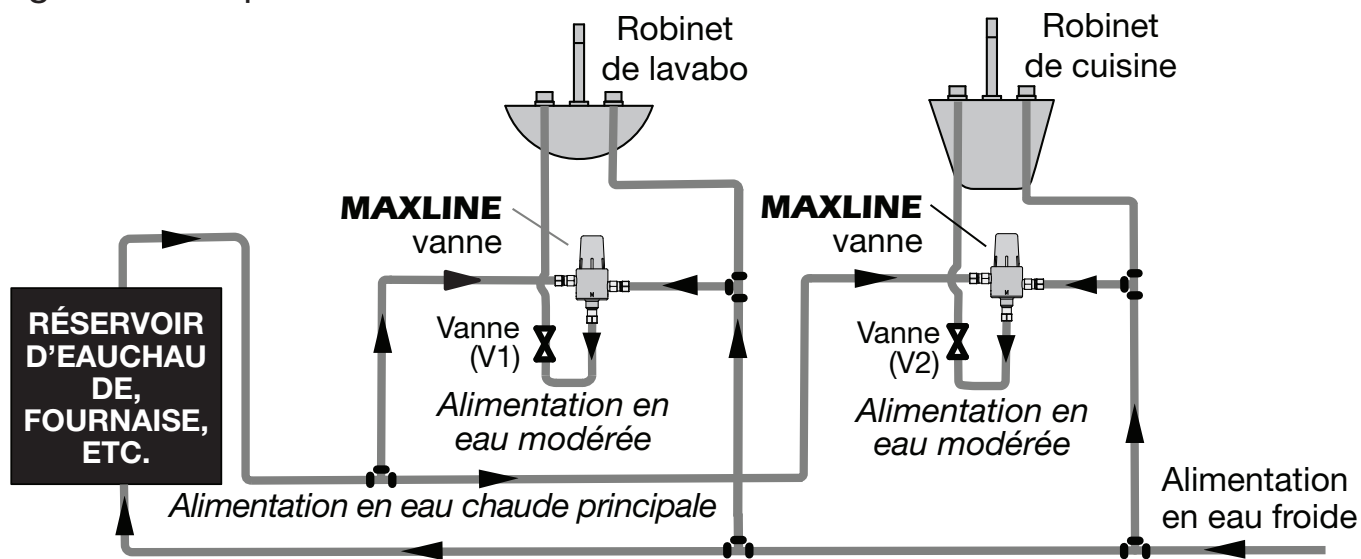
Diagramme du point d'utilisation
