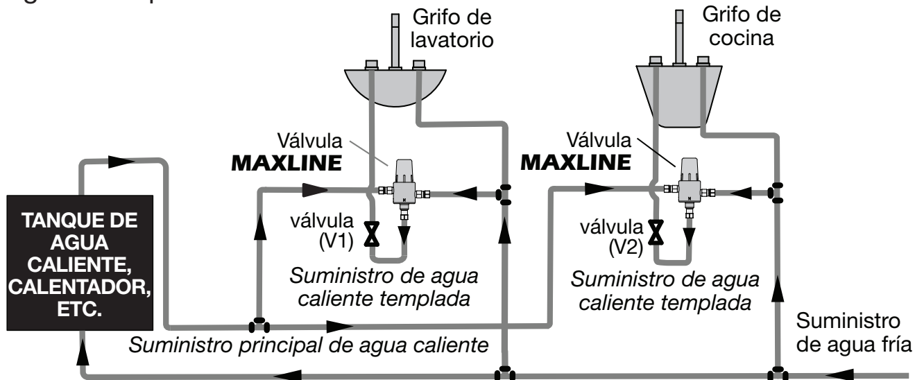
Diagrama de punto de uso
